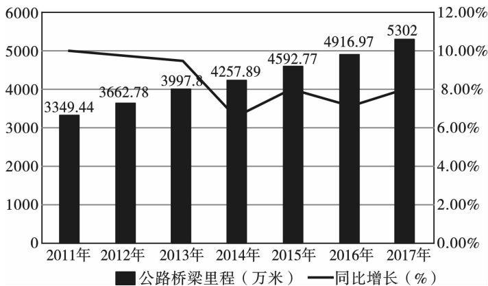
图1 2011~2017年我国公路桥梁里程增长
