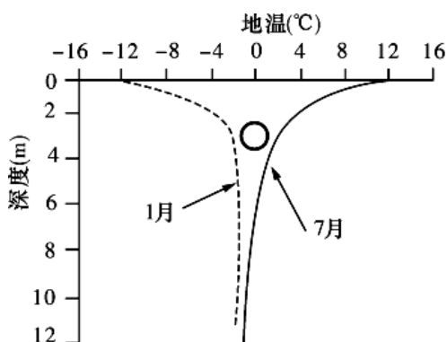
a图 漠大线加格达奇观测站地温变化图
