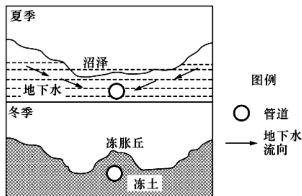
b图 季节性冻胀丘形成剖面示意图
