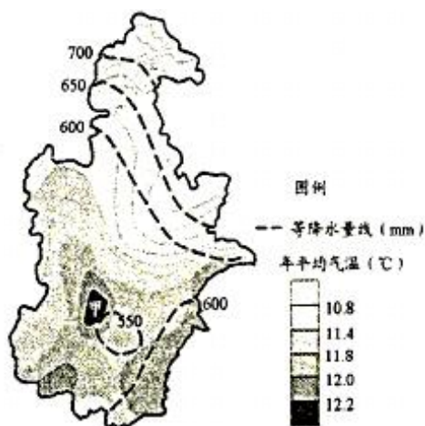
图 2 天津市年平均气温和降水分布图
